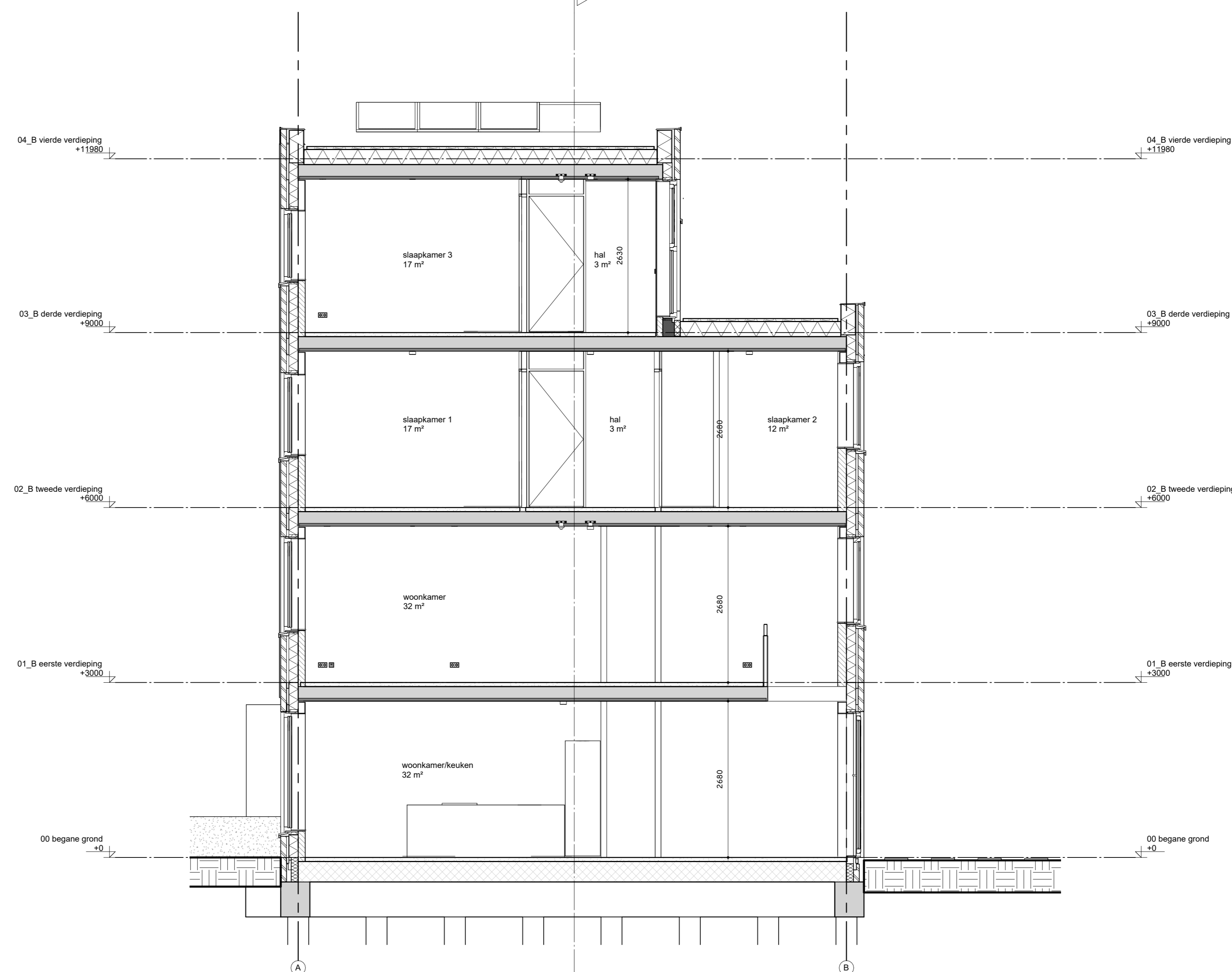
optie_vide doorsneden
