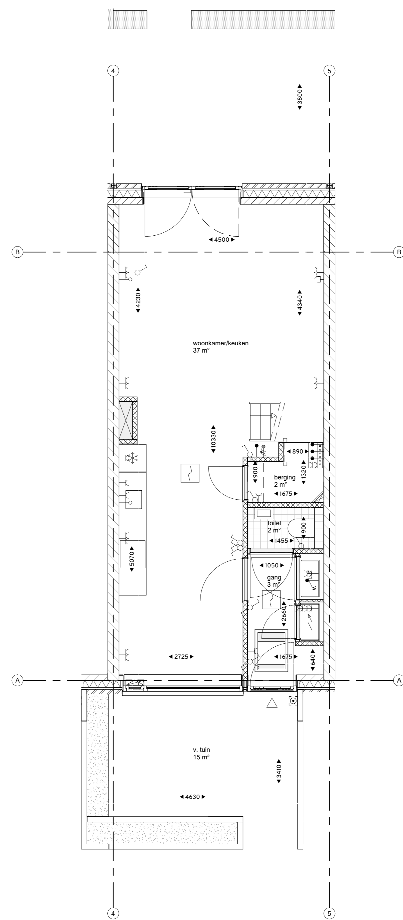
optie_uitbouw 1.2 begane grond
