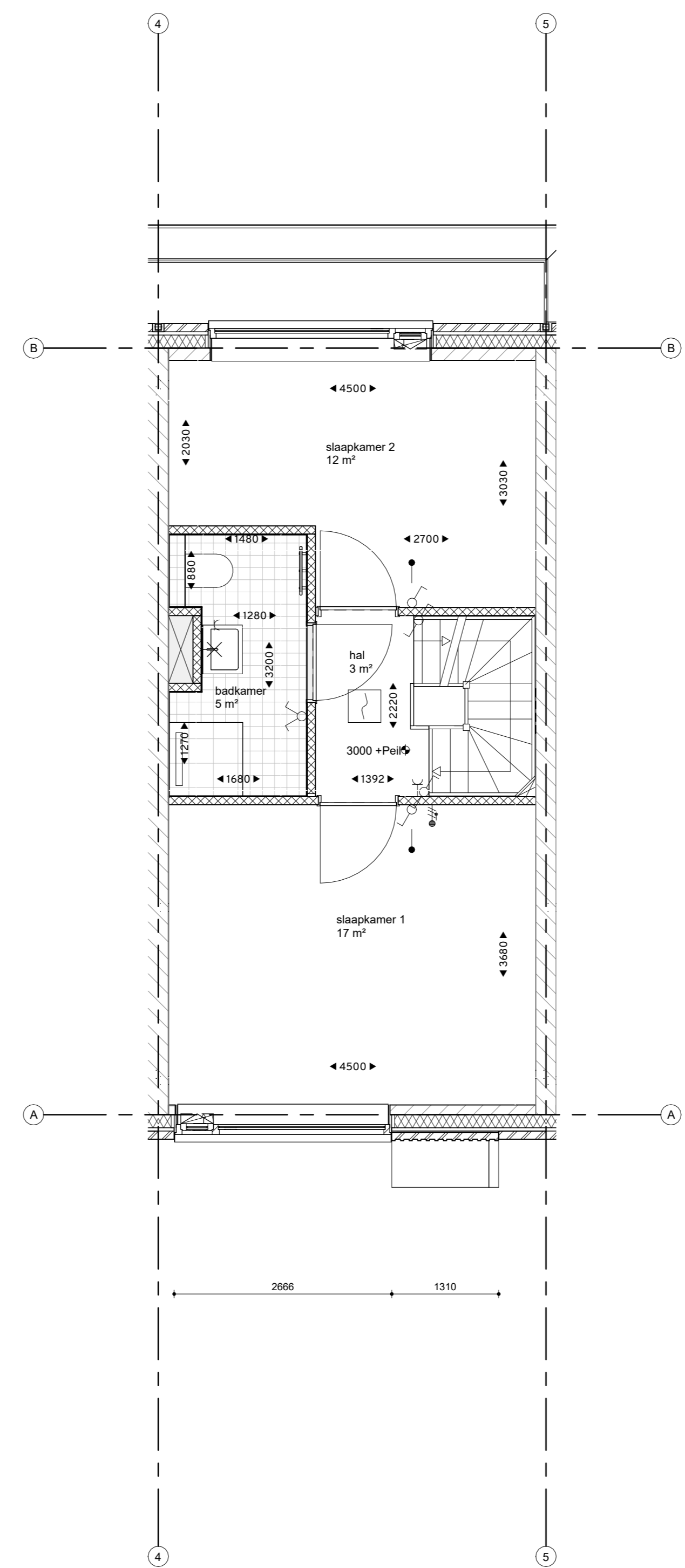
optie_uitbouw 1.2 eerste verdieping
