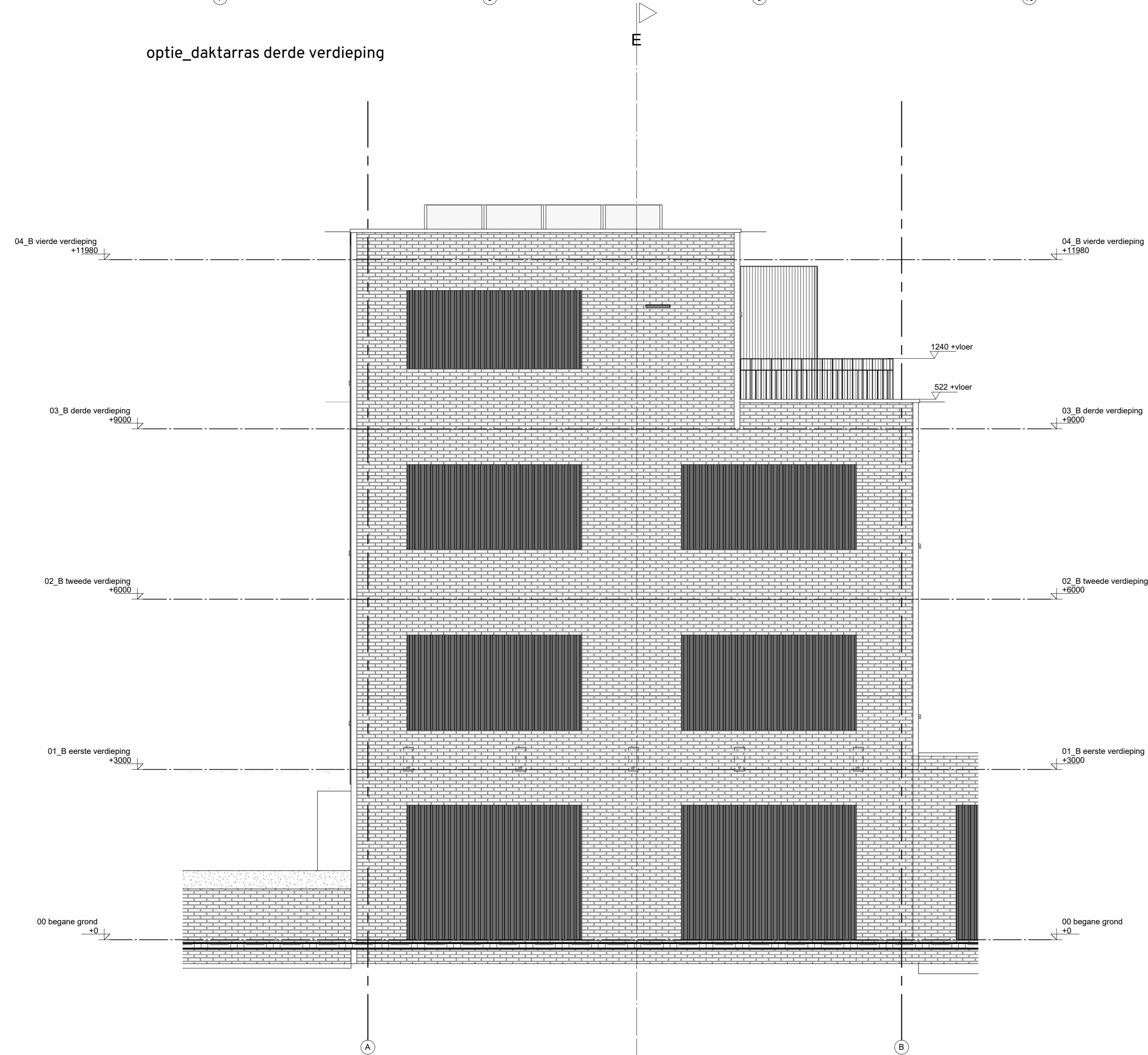
optie_dakterras gevel oost
