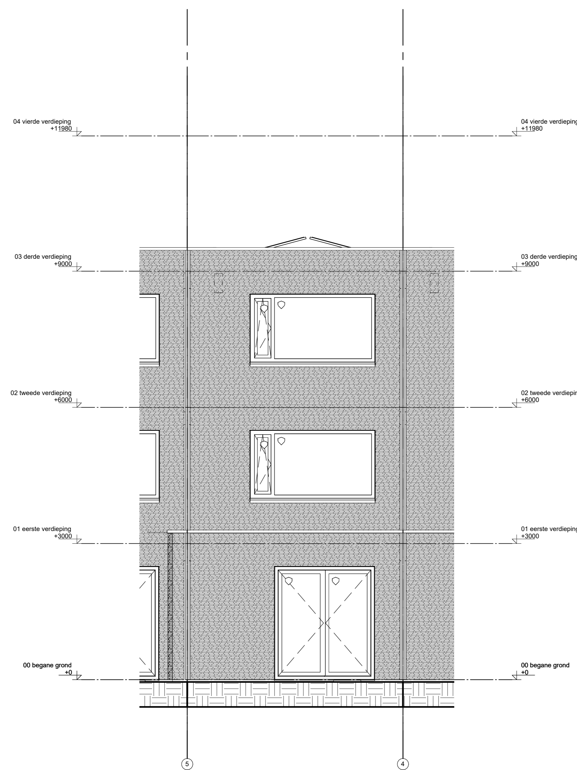
optie_uitbouw 1.2 gevel noord
