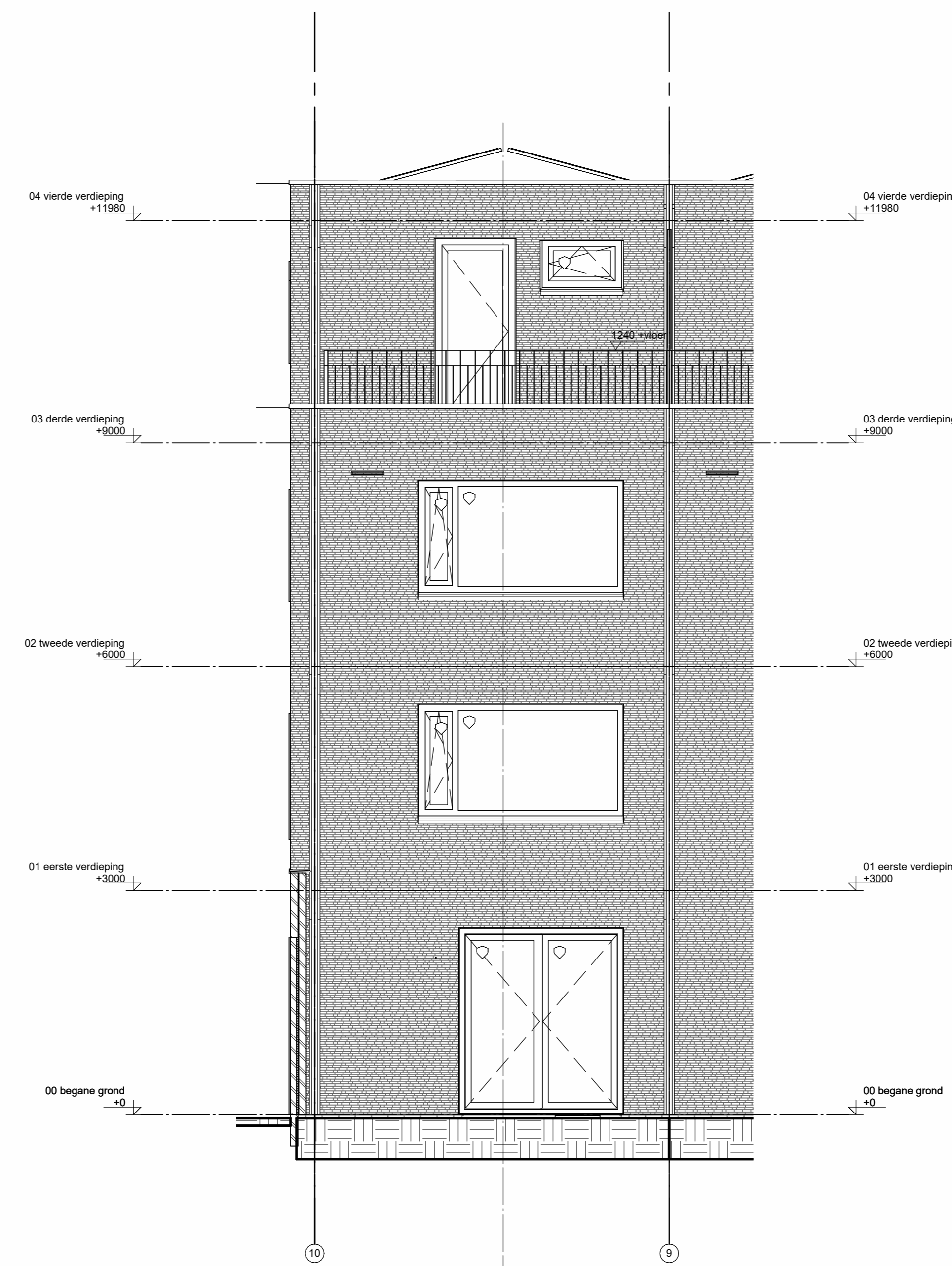
optie_dakterras gevel noord
