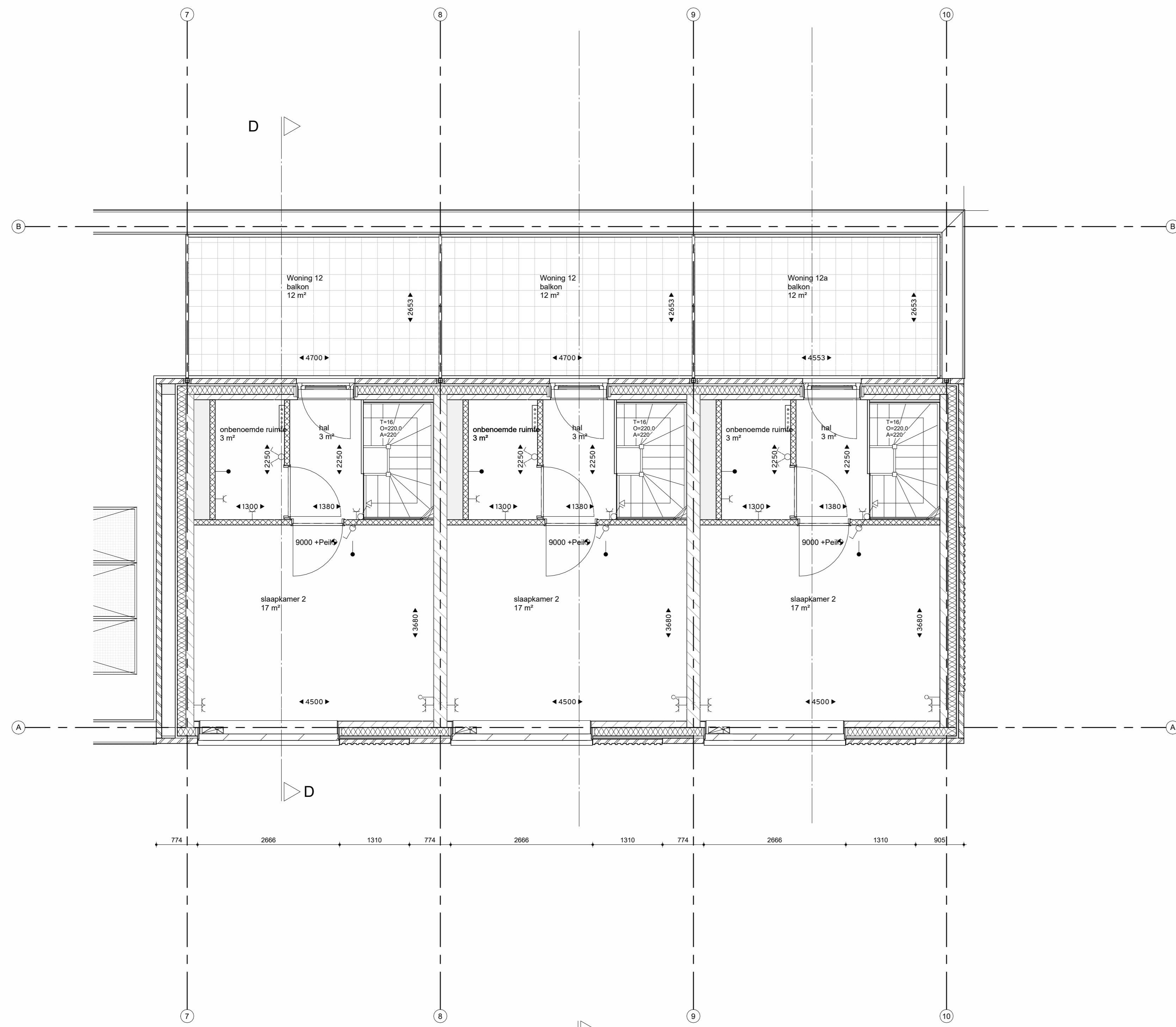
optie_dakterras derde verdieping
