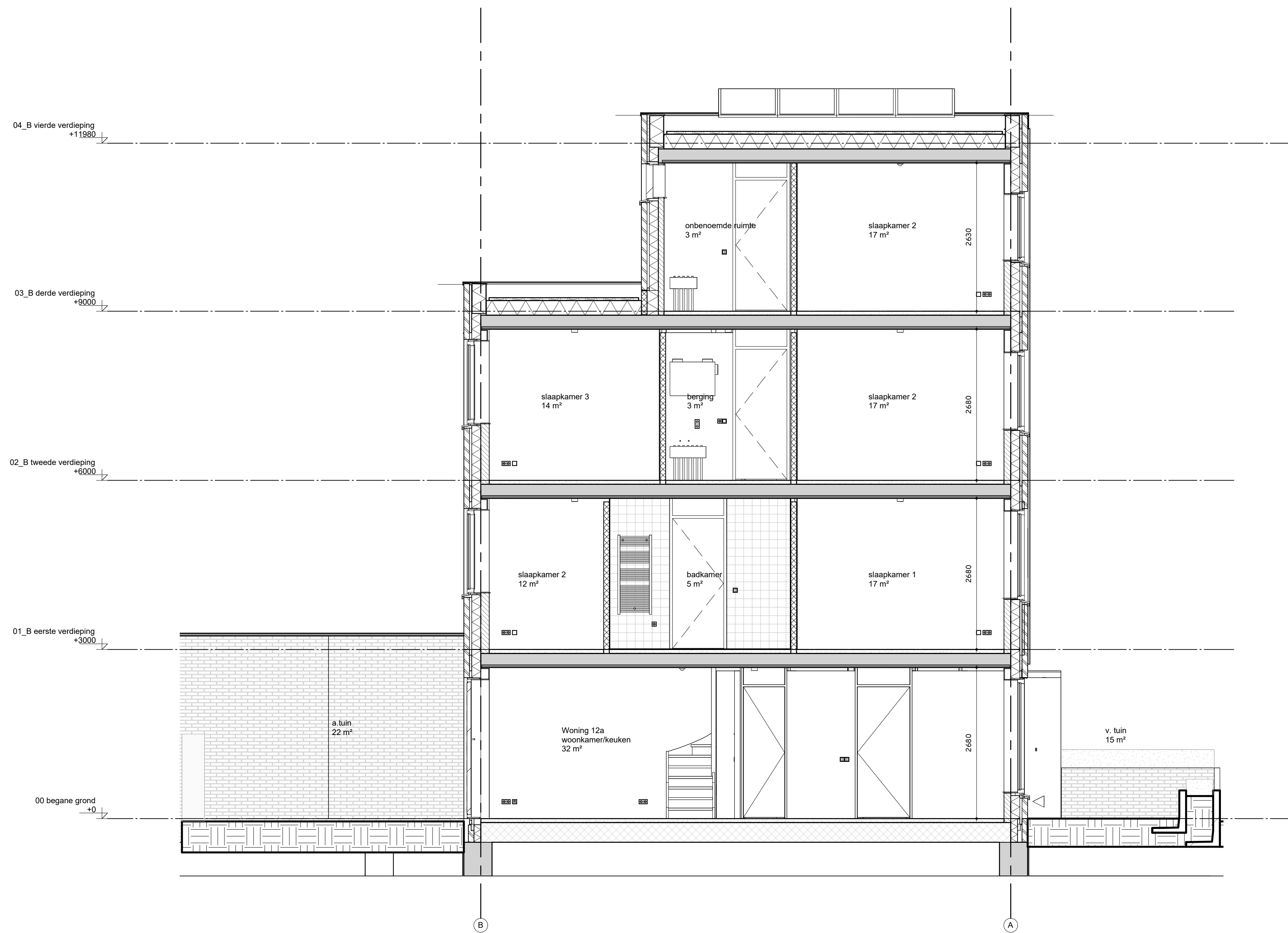
bnr. 009 doorsnede
