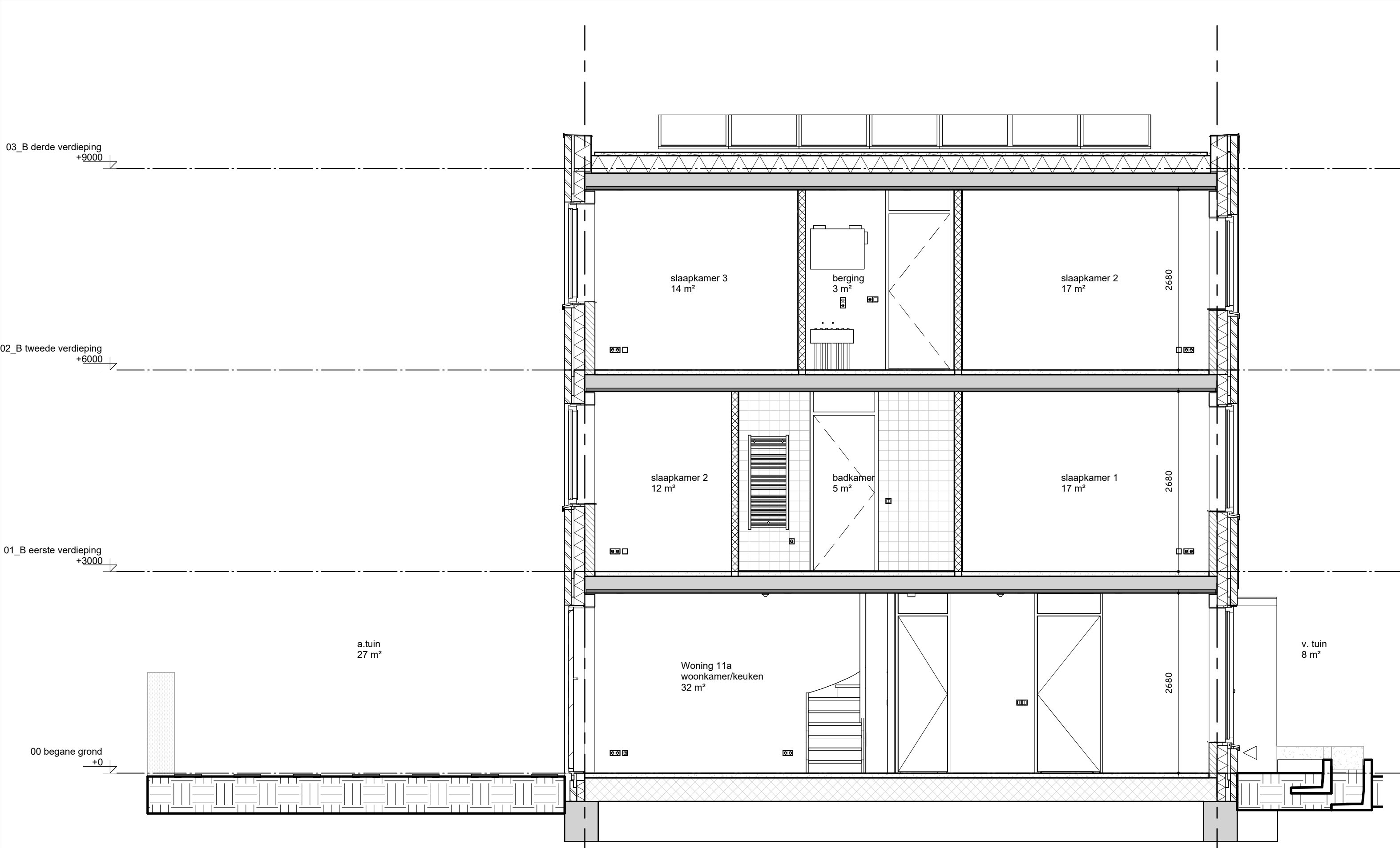
bnr. 010 doorsnede
